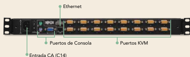
B020-016-17-IP (frente/atrás)
