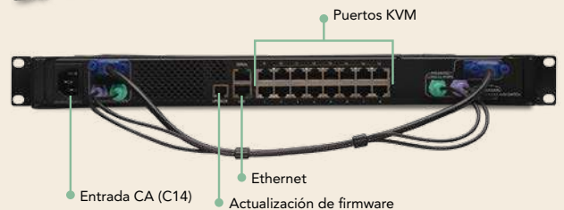
B070-016-19-IP (frente/atrás)
